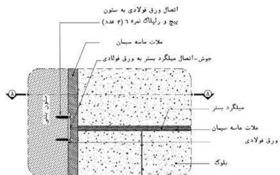
Det.1
