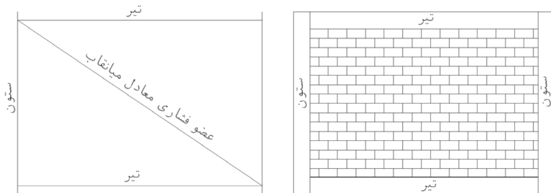
الف) دیوار با عملکرد میانقابی (ب) مدل قاب میانپیر
